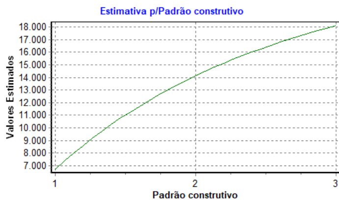
Gráfico 6 – Estimativa para padrão construtivo
