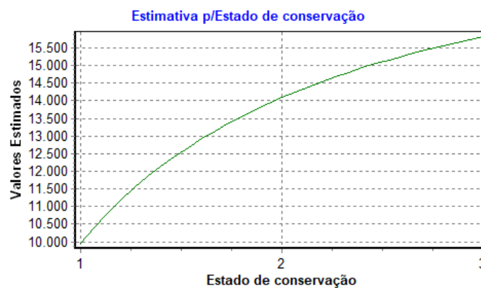
Gráfico 7 – Estimativa para estado de conservação
