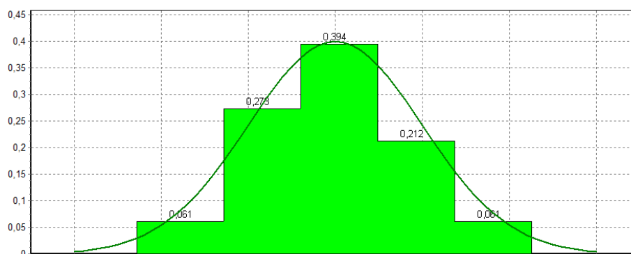
Gráfico 3 – Normalidade dos Resíduos
