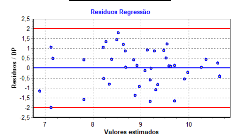
Gráfico 2 - Resíduos da Regressão Linear
