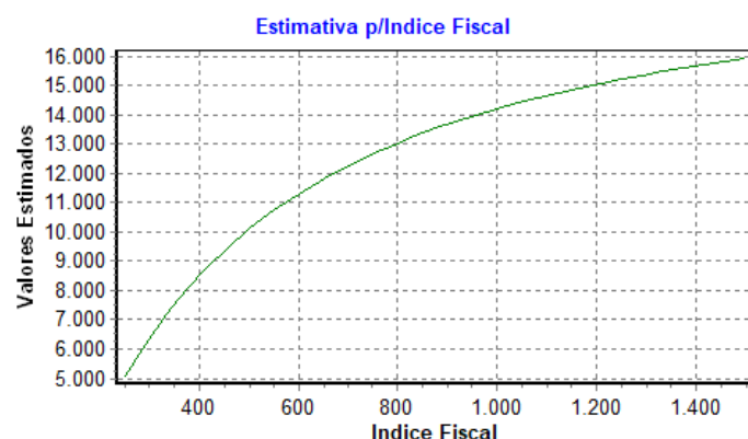
Gráfico 5 – Estimativa para índice fiscal
