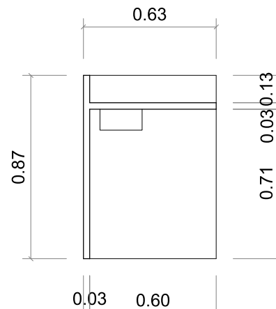
VISTA CORTE esc.: 1:25
