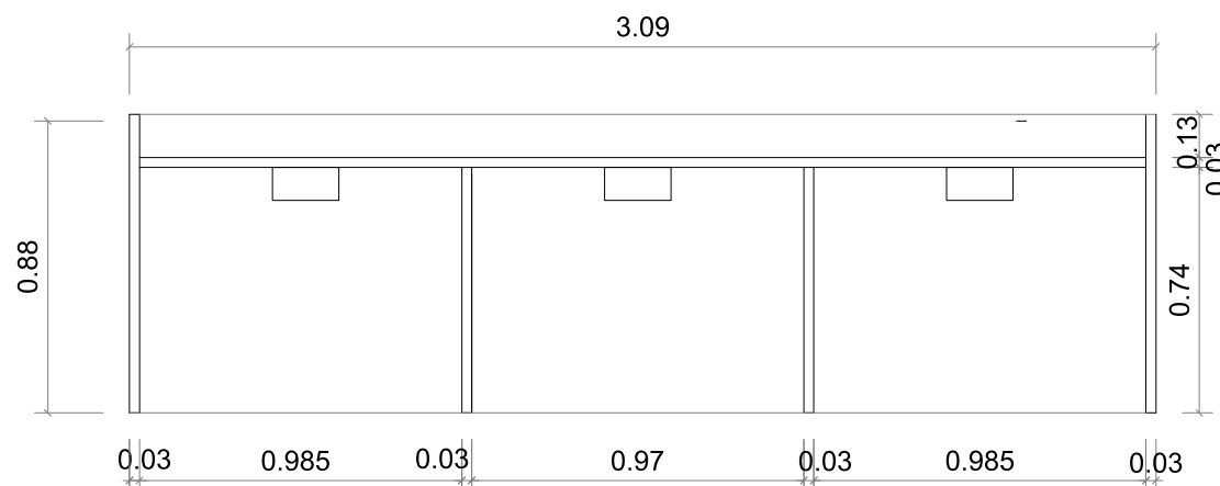
VISTA POSTERIOR esc.: 1:25
