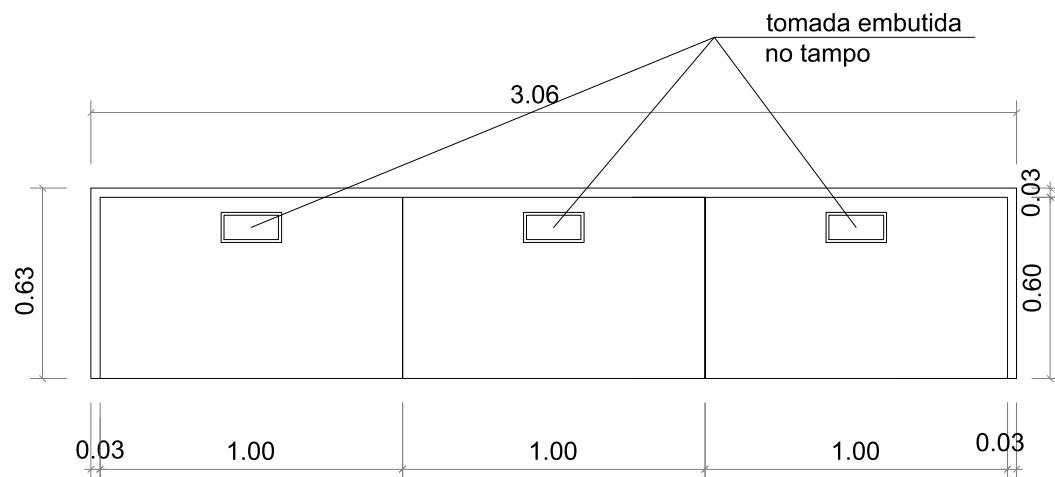
VISTA SUPERIOR esc.: 1:25
