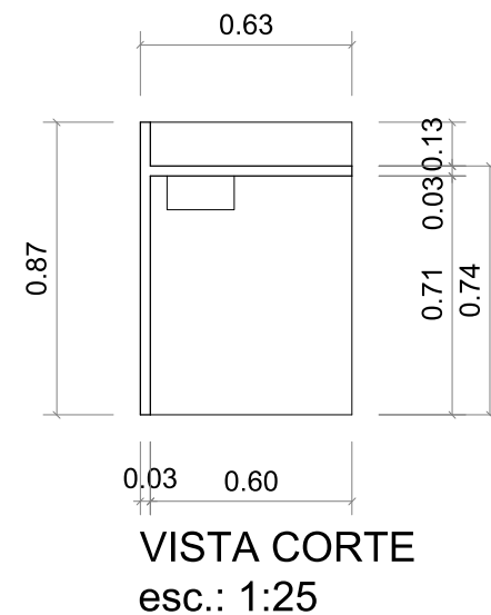
TOMADA EMBUTIDA IMAGEM ILUSTRATIVA
