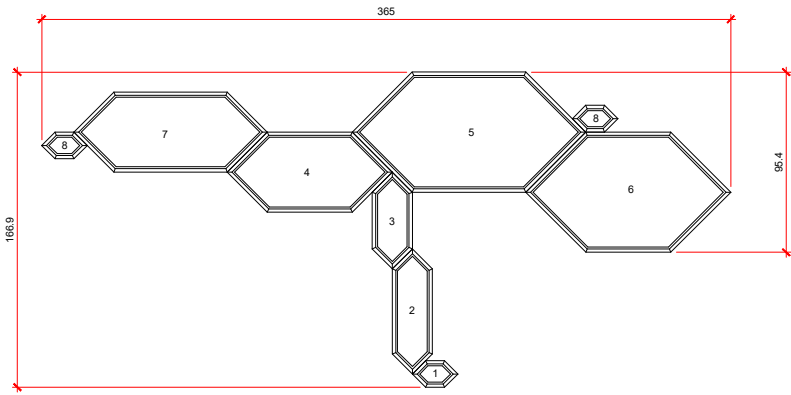
PLANTA BAIXA GERAL ESC. 1:20
