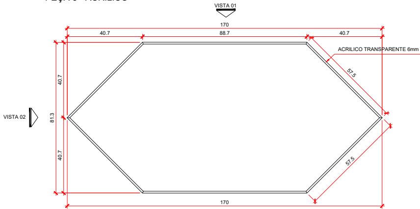
PLANTA BAIXA ESC. 1:10
