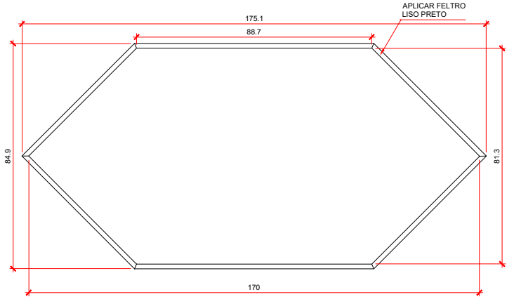
PLANTA INFERIOR ESC. 1:10
