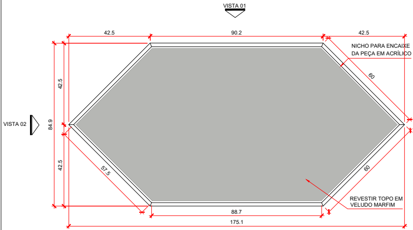
PLANTA BAIXA ESC. 1:10
