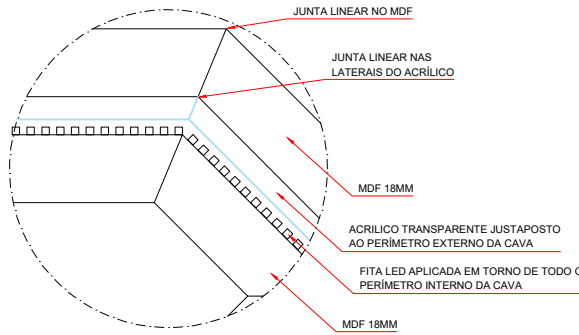
PLANTA ESC. 1:1
