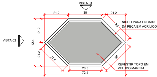
PLANTA BAIXA ESC. 1:10
