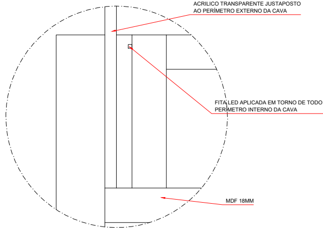
CORTE ESC. 1:1
