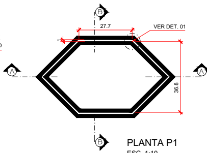
PLANTA P1 ESC. 1:10
