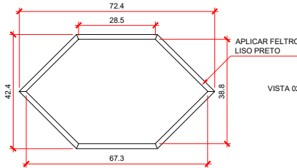
PLANTA INFERIOR ESC. 1:10
