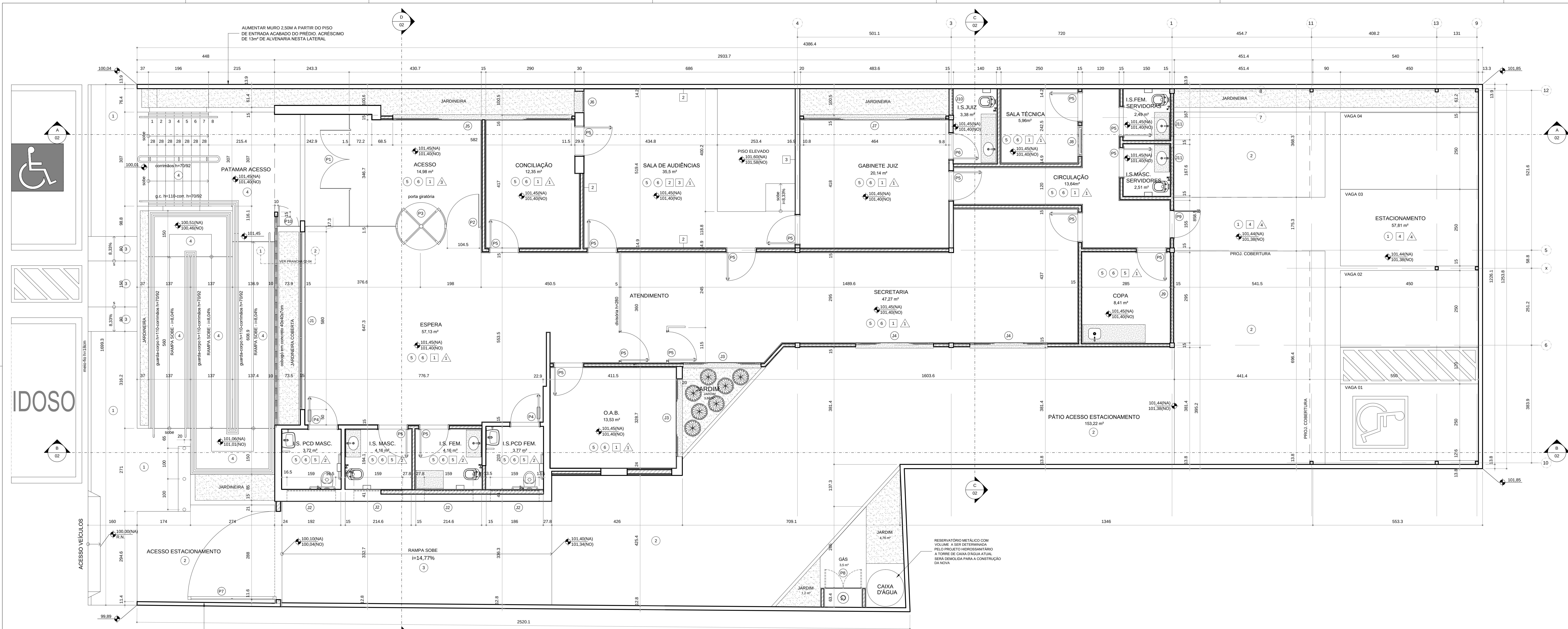
PLANTA TÉRREO E ESTACIONAMENTO
