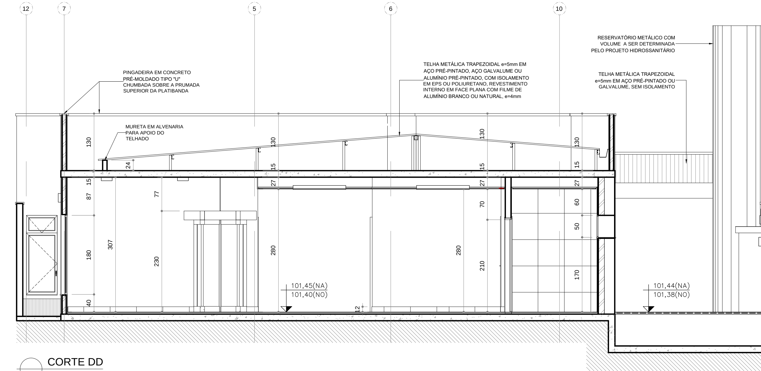
CORTE DD ESCALA: 1/50
