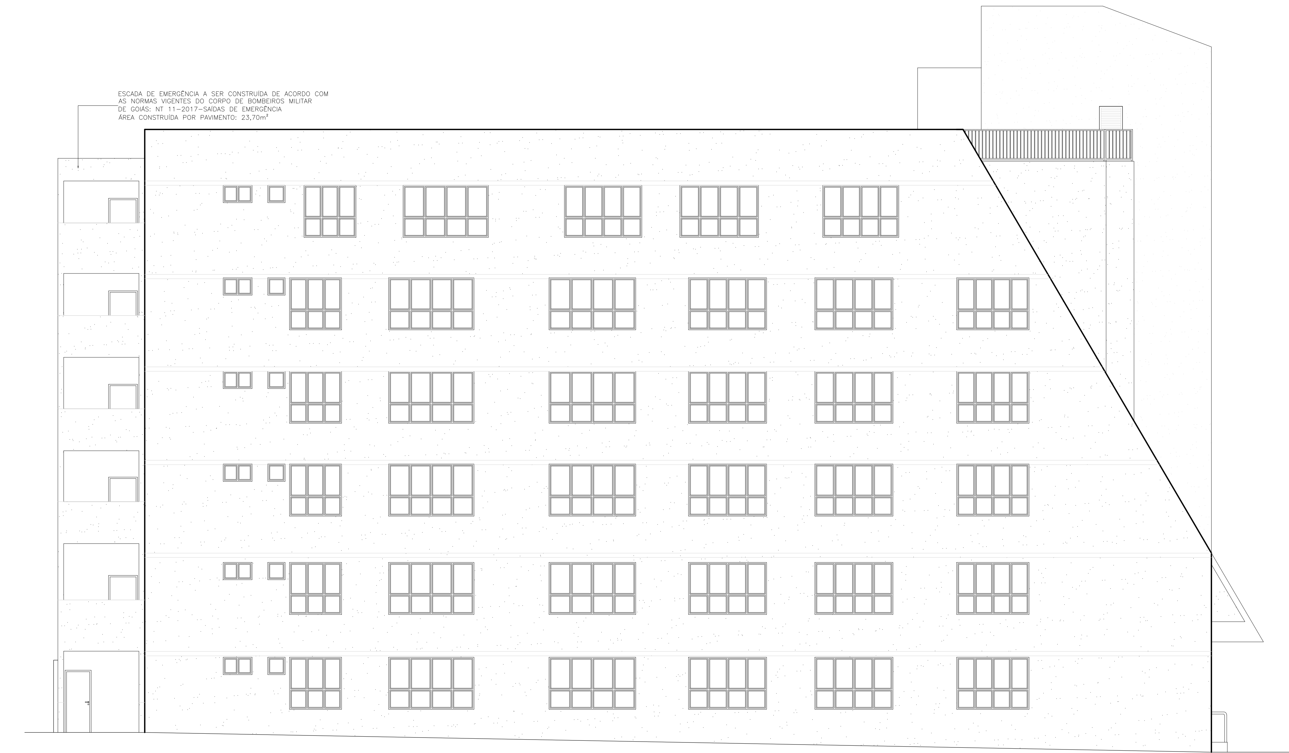
FACHADA LATERAL ESQUERDA ESCALA: 1/75
