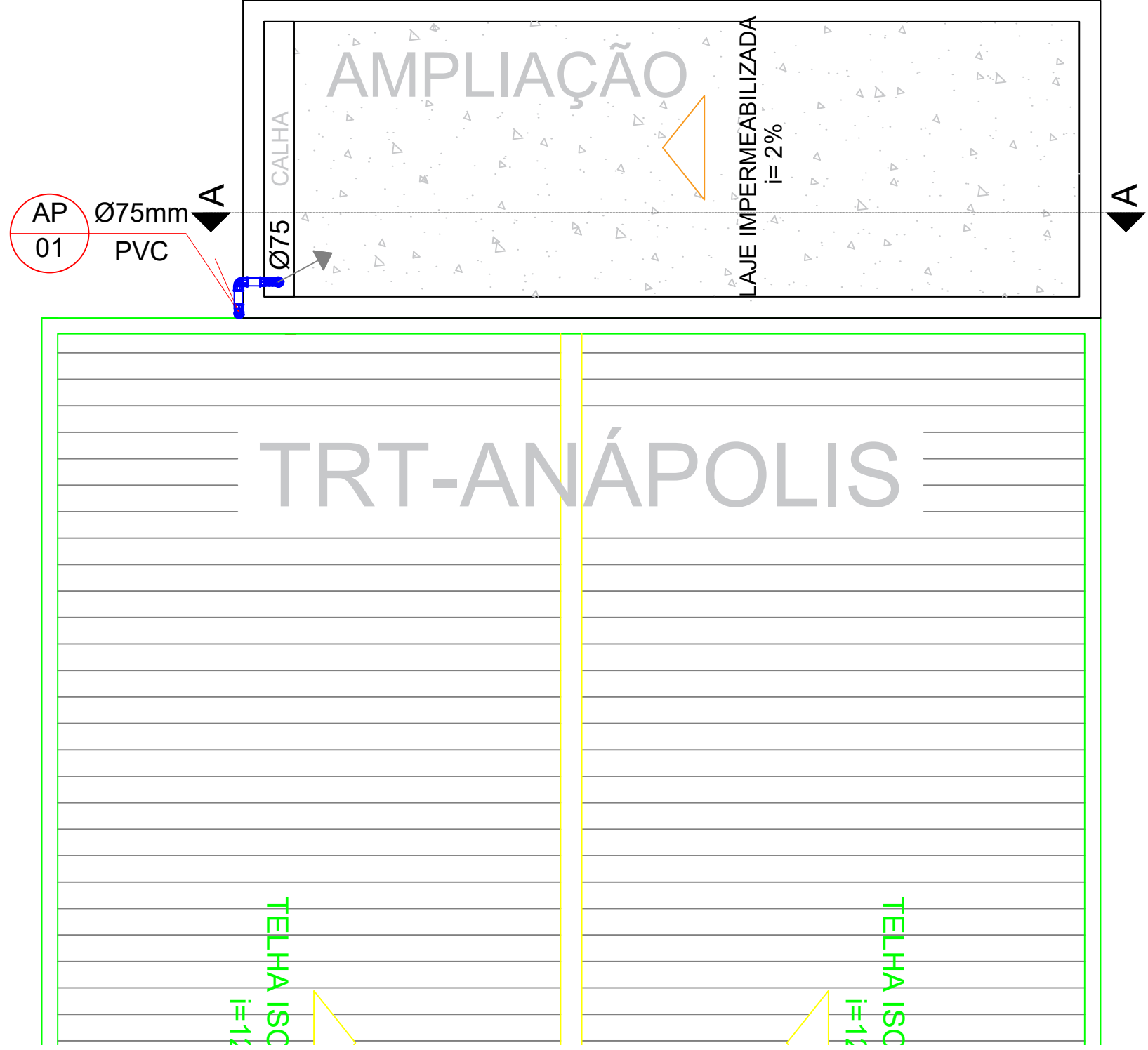
PLANTA DE COBERTURA - AMPLIAÇÃO ESC: 1/50
