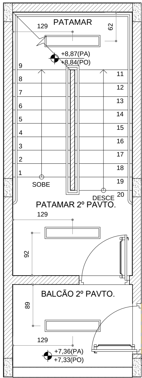
PLANTA 2º PAVIMENTO ESCALA: 1/50
