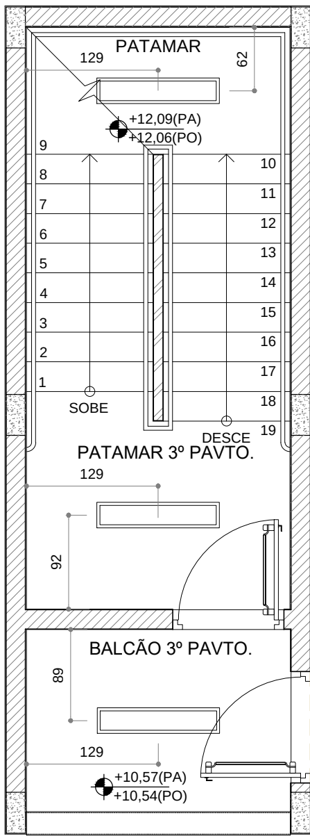
PLANTA 3º PAVIMENTO ESCALA: 1/50
