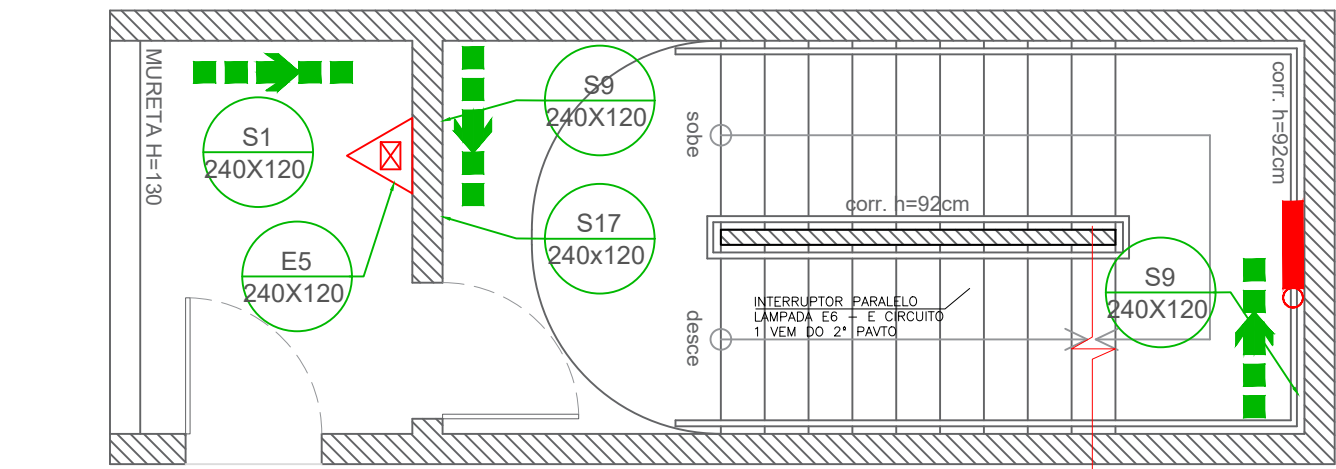
3º PAVIMENTO
