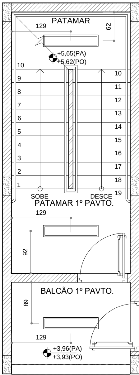
PLANTA 1º PAVIMENTO ESCALA: 1/50
