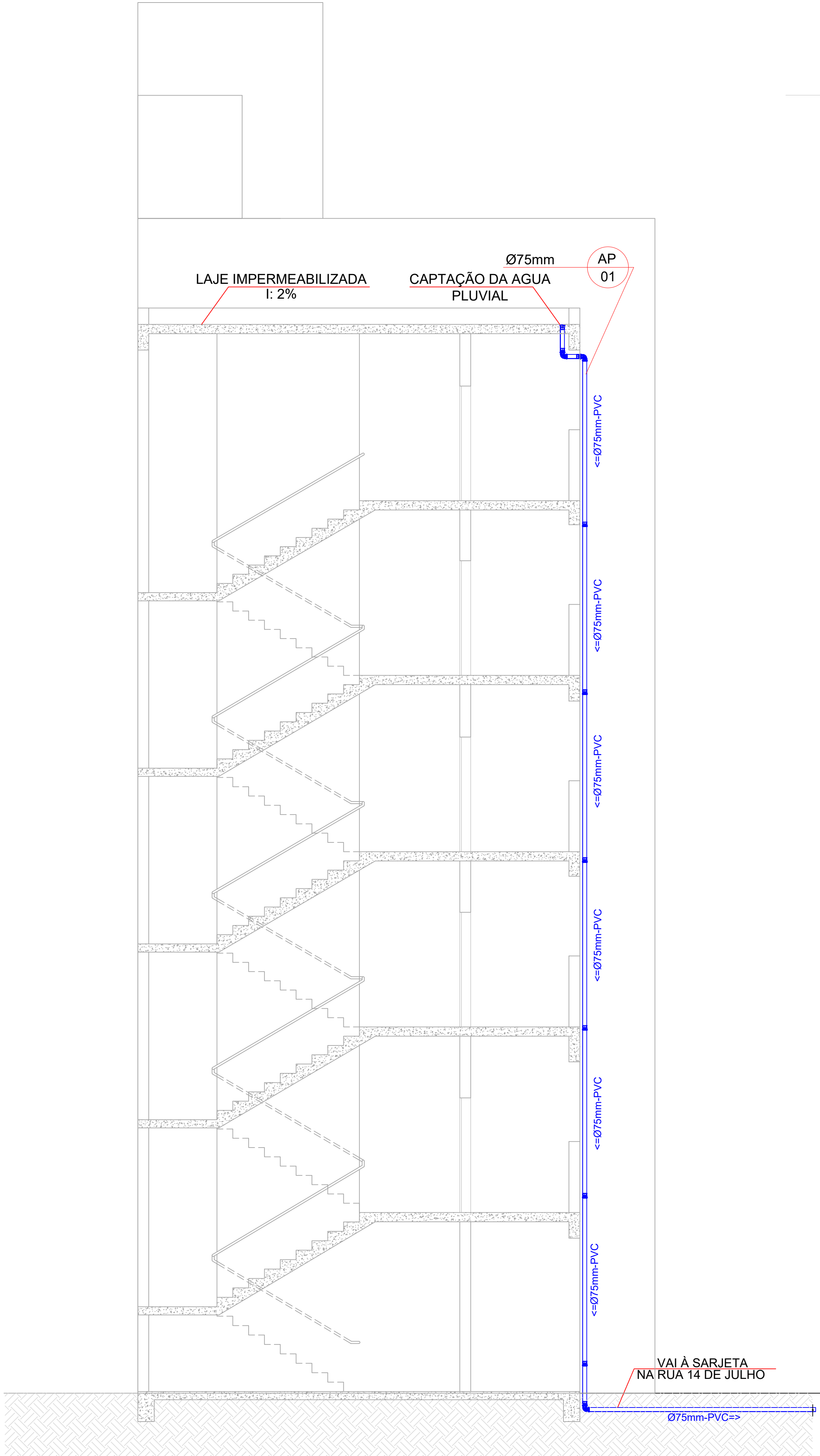
CORTE ESC: 1/50
