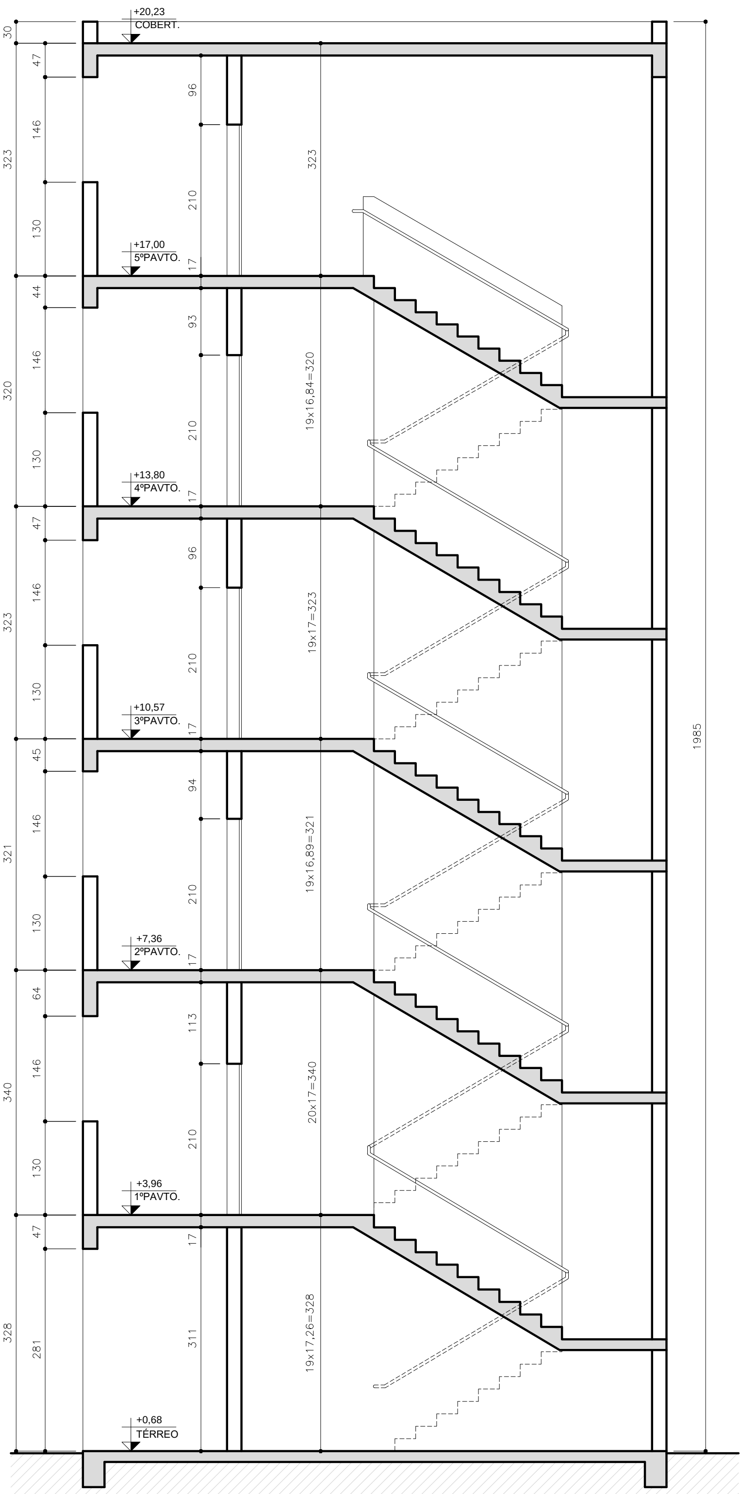
CORTE GH ESCALA: 1/50
