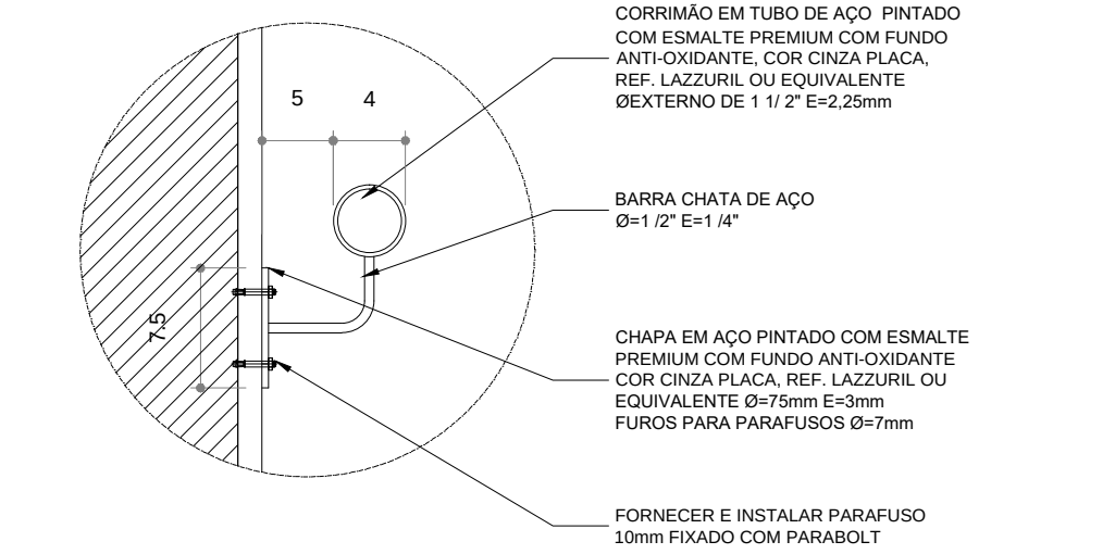
DETALHE FIXAÇÃO CORRIMÃO NA ALVENARIA ESCALA: 1/5
