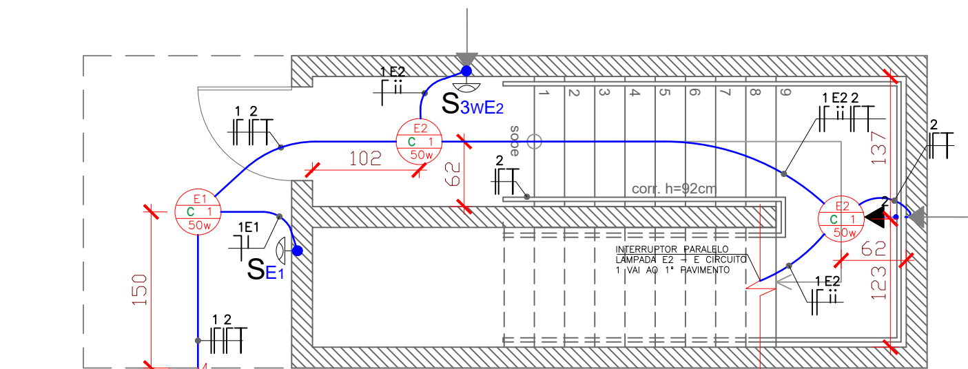
TÉRREO ESC:1/75
