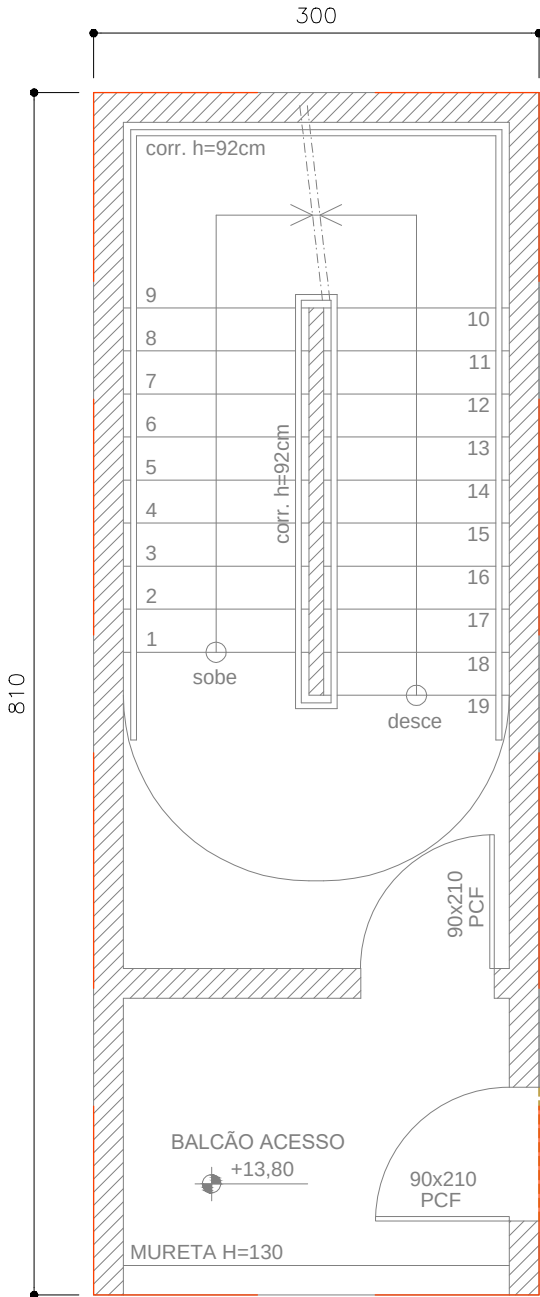
PLANTA ESCADA EMERGÊNCIA ESCALA: 1/50 ÁREA: 24,30m²
