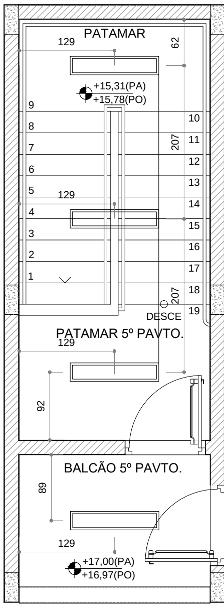
PLANTA 5º PAVIMENTO ESCALA: 1/50
