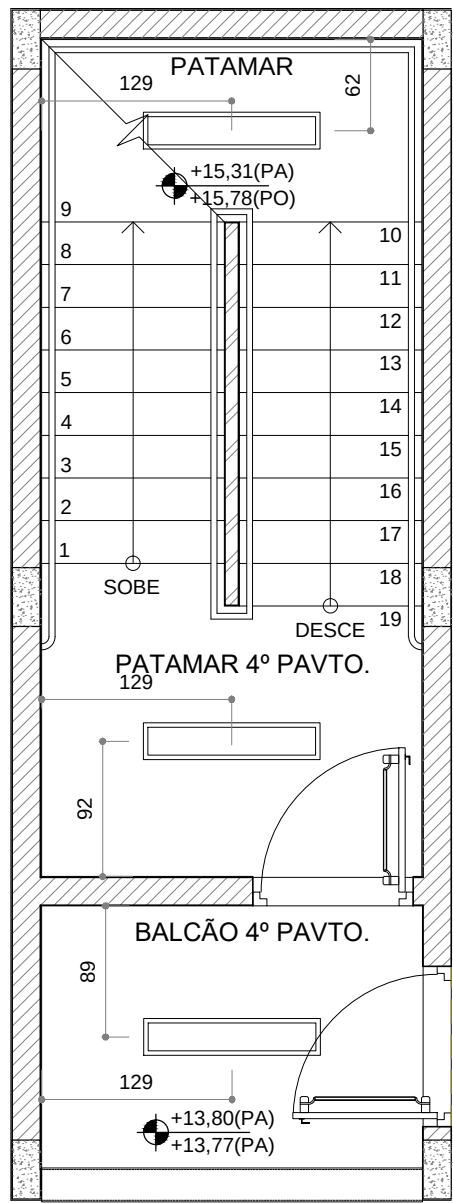
PLANTA 4º PAVIMENTO ESCALA: 1/50
