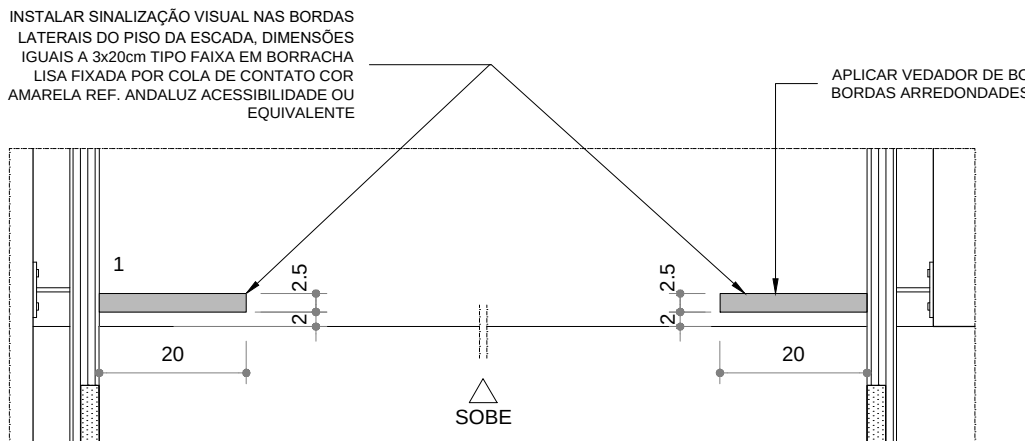
DETALHE PADRÃO SINALIZAÇÃO VISUAL PISO ESCALA: 1/10
