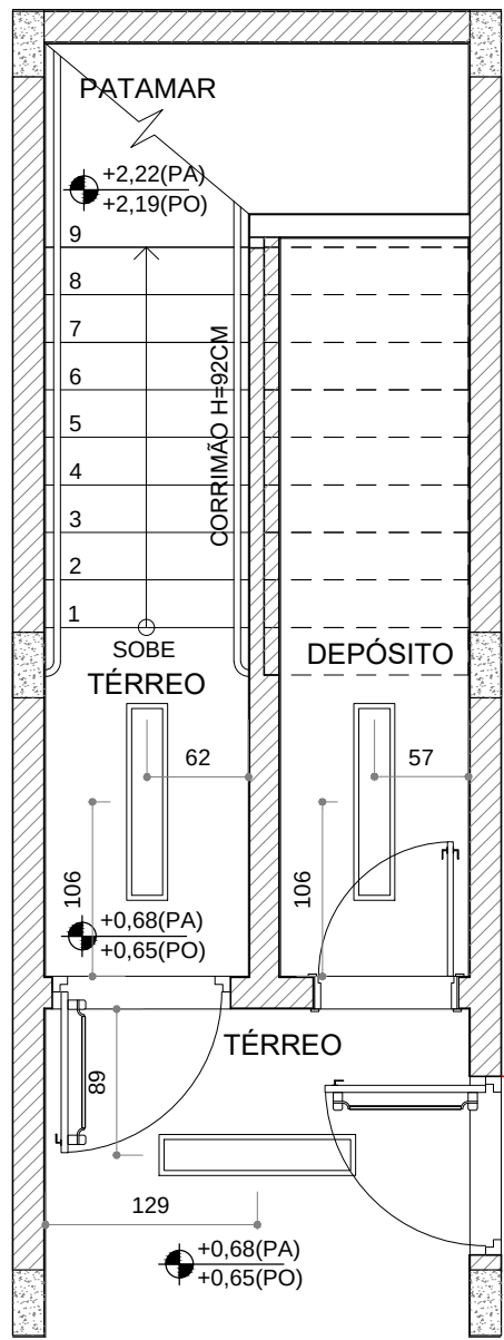
PLANTA TÉRREO ESCALA: 1/50
