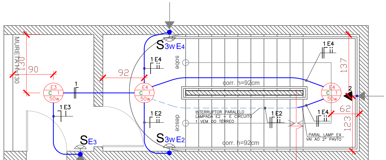
1º PAVIMENTO ESC:1/75
