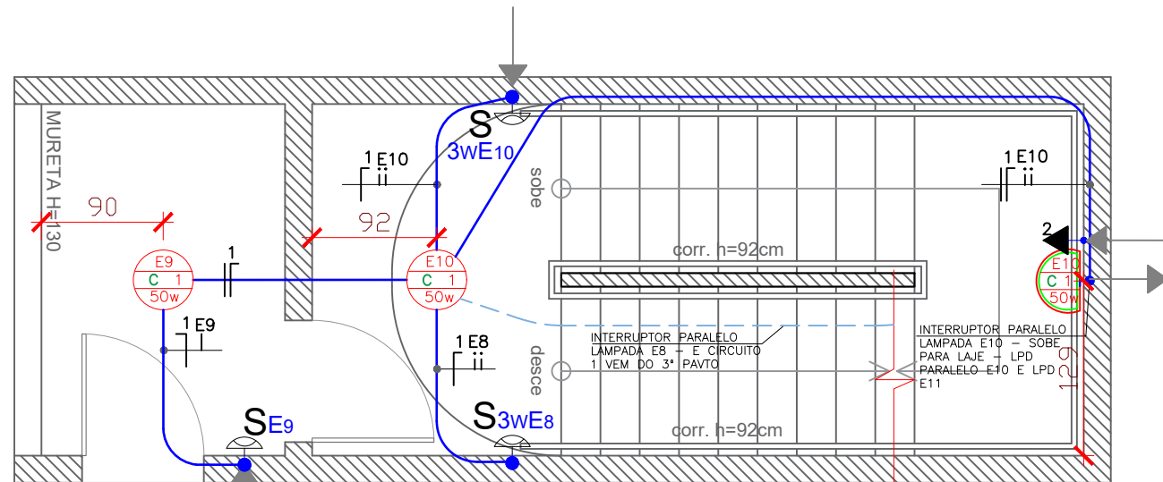
4º PAVIMENTO ESC:1/75
