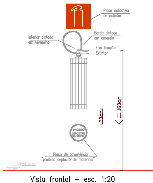
Observação extintores
