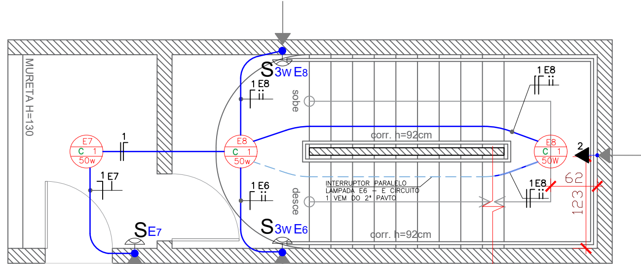
3º PAVIMENTO ESC:1/75
