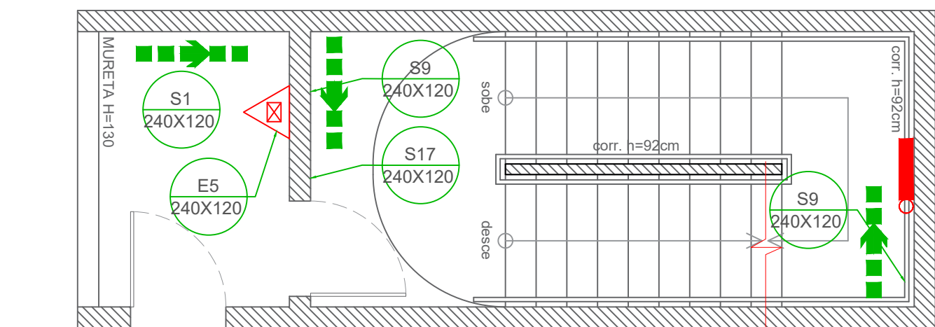
2º PAVIMENTO
