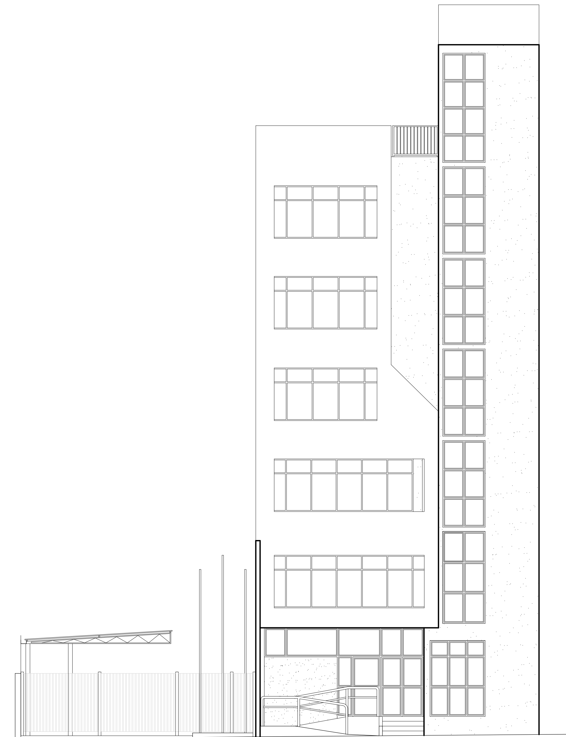
FACHADA FRONTAL RUA 14 DE JULHO ESCALA: 1/75
