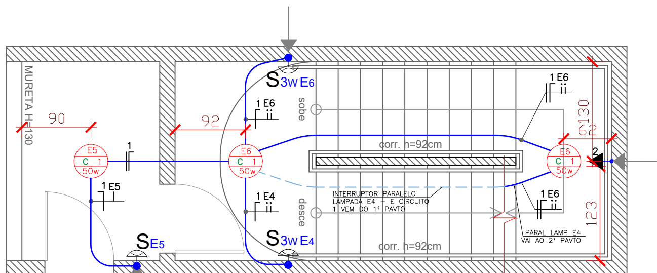
2º PAVIMENTO ESC:1/75
