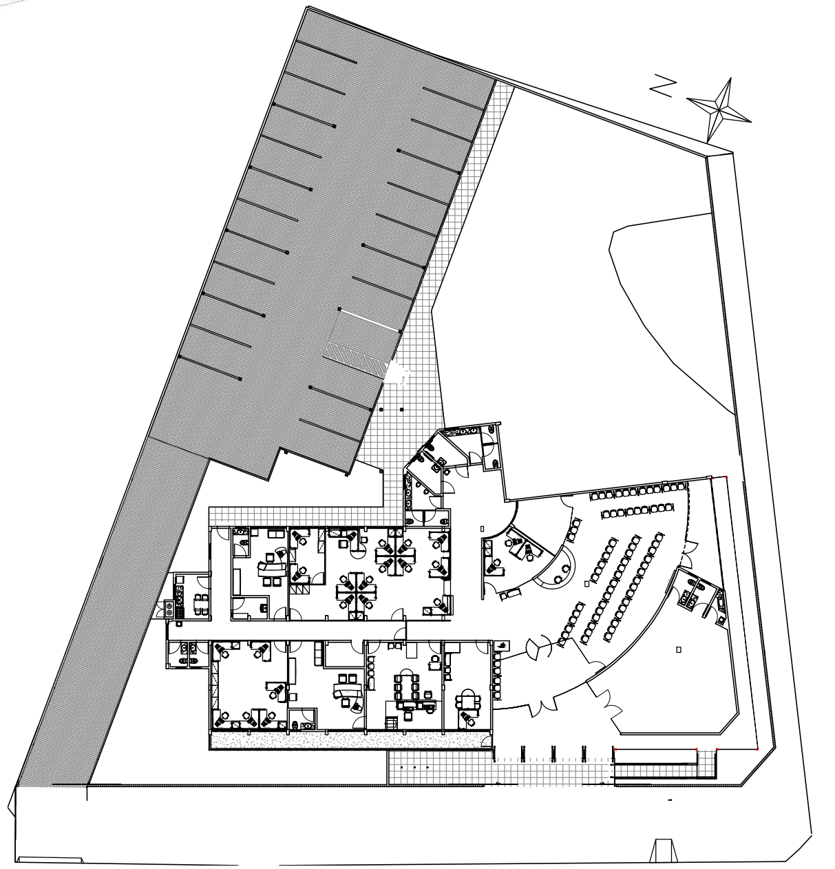
2) PLANTA LAYOUT ESC. 1: 200
