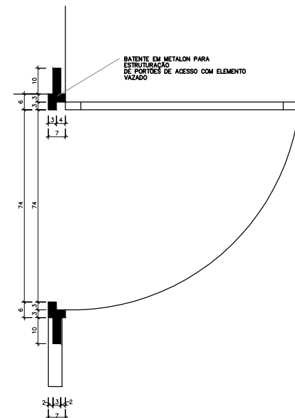
ELEMENTO VAZADO / DETALHE ESTRUTURAÇÃO PORTÃO DE ACESSO ESC. 1: 10
