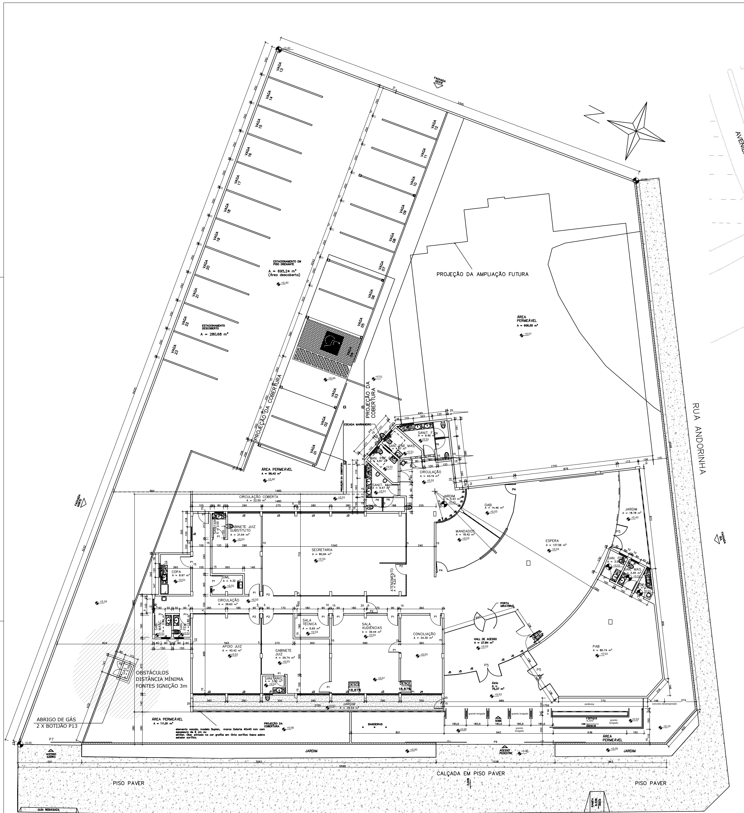
1) PLANTA PAVIMENTO TERREO ESC. 1: 100
