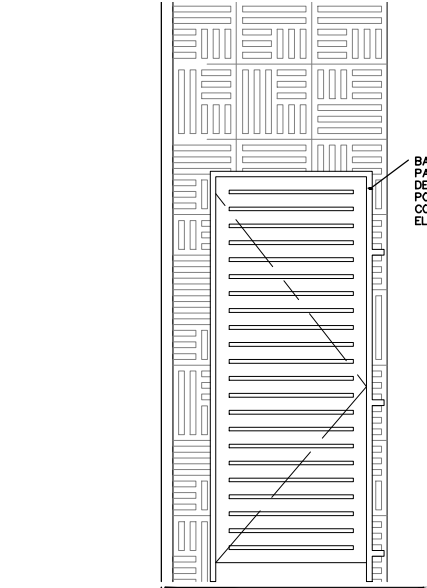
3) VISTA BATENTE EM METALON PARA ACESSO PAREDE ELEMENTO VAZADO ESC. 1: 20
