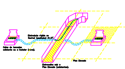
DETALHE DE INSTALAÇÃO DE NOVAS TOMADAS
