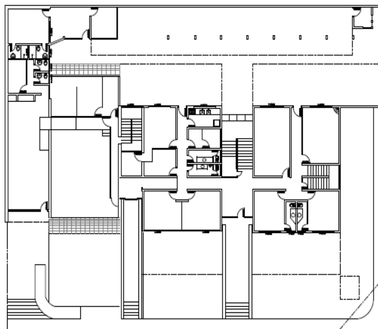
ANEXO PORTUGAL PLANTA BAIXA PAVTO TERREO - ATUAL esc. 1:250
