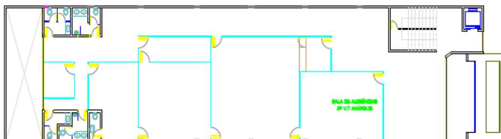
F.T. ANÁPOLIS PLANTA BAIXA 2º PAVTO - ATUAL esc.1:200
