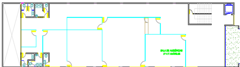
F.T. ANÁPOLIS PLANTA BAIXA 1º PVTO - ATUAL esc.1:200
