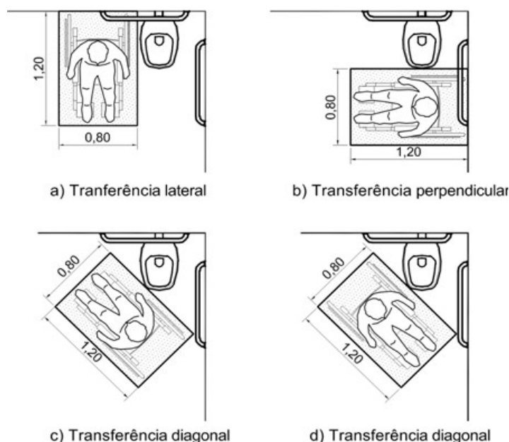
Área de Transferência em Bacias Sanitárias Exemplo NBR9050:2004
