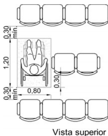
Espaço P.C.R. Fileira Intermediária Exemplo NBR9050:2004
