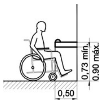
VISTA LATERAL
