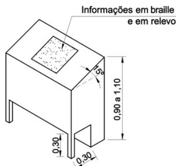
Superfície Inclinada com Informações Táteis Exemplo NBR9050:2004
