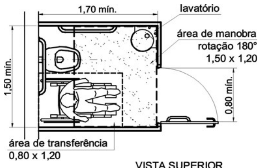
Boxe para Bacia Sanitária - Medidas Mínimas Exemplo NBR9050:2004
