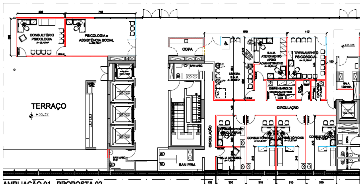
AMPLIAÇÃO 01 - PROPOSTA 02 ASSISTÊNCIA MÉDICA, PSICOLOGIA e ASSISTÊNCIA SOCIAL
