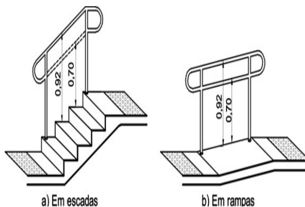
Corrimãos em degraus - Exemplo NBR9050:2004
