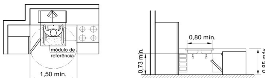
Copas / Cozinhas - Exemplo NBR9050:2004
