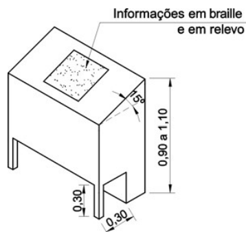
Superfície Inclinada com Informações Táteis Exemplo NBR9050:2004
