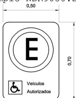
Sinalização Vertical de Vagas em Espaço Interno Exemplo NBR9050:2004
