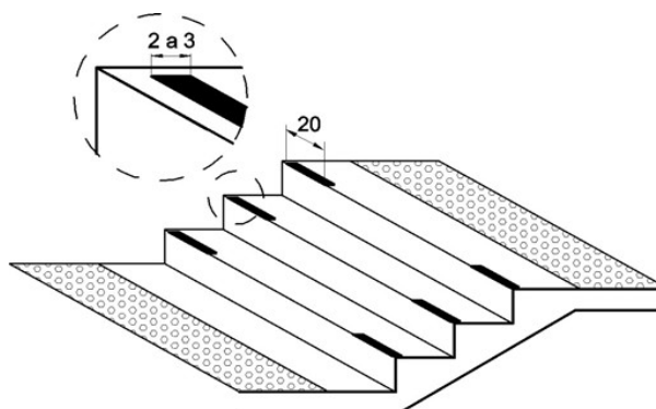
Sinalização visual de degraus - Exemplo NBR9050:2004
