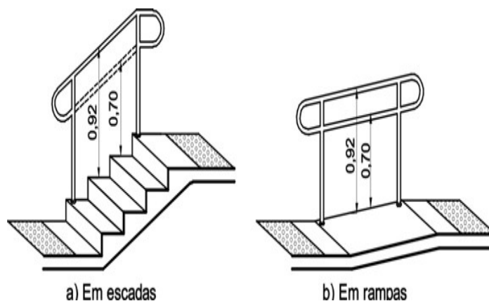
Corrimãos em rampas - Exemplo NBR9050:2004
