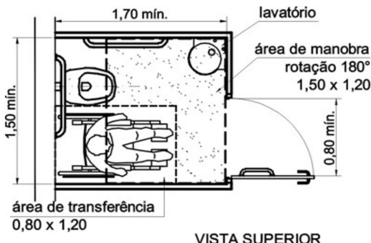
Boxe para Bacia Sanitária Medidas Mínimas Exemplo NBR9050:2004
