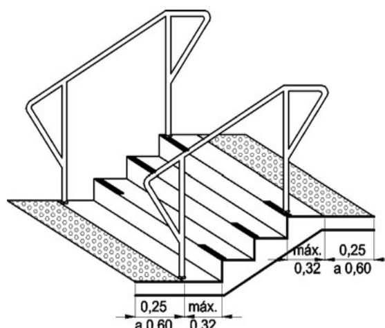
Sinalização Tátil de Alerta em Escadas Exemplo NBR9050:2004
