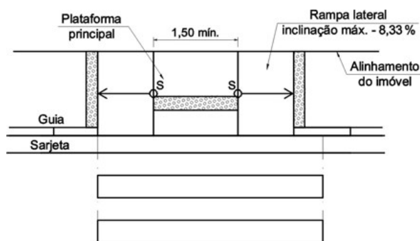
Rebaixamento de Calçadas - Exemplo NBR9050:2004
