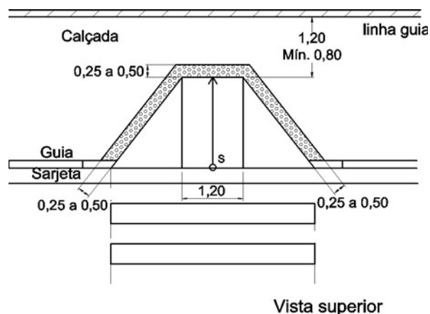
Sinalização Tátil de Alerta em Rebaixamento de Calçadas Exemplos NBR9050:2004
