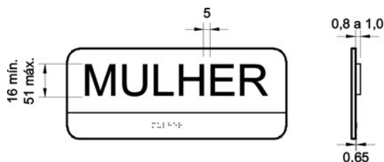
Ampliação Sinalização Portas - Exemplo NBR9050:2004
