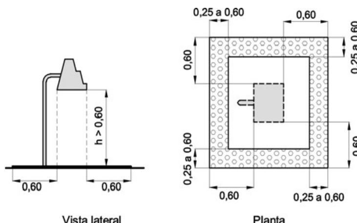
Sinalização tátil de alerta - obstáculos suspensos Exemplo NBR9050:2004
