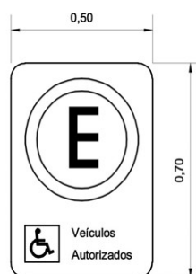
Sinalização vertical de vaga para PNE Exemplo NBR9050:2004
