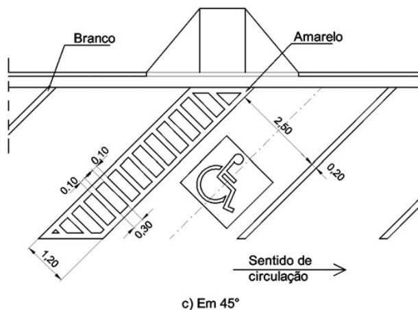
Sinalização horizontal de vaga para PNE Exemplo NBR9050:2004
