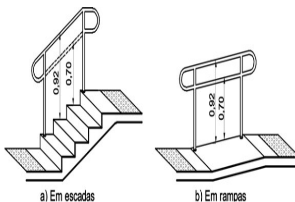
Corrimãos em degraus - Exemplo NBR9050:2004
