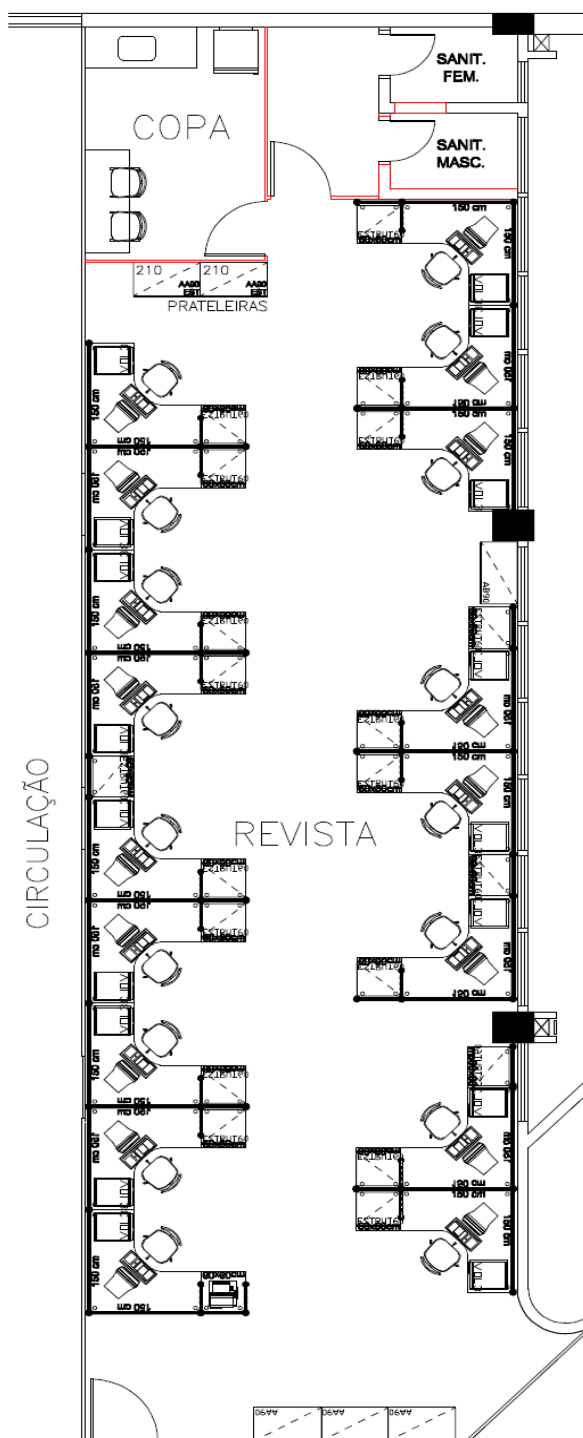
ED. SEDE - 5º PAVTO. LAY-OUT / RECURSO DE REVISTA Esc: 1:100
