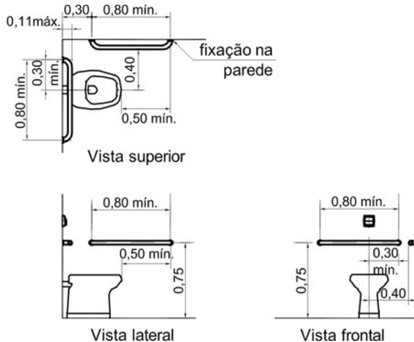
Bacia Sanitária - Barra de apoio lateral e de fundo Exemplo NBR9050:2004
