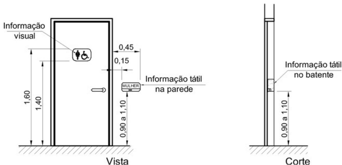
Sinalização portas - exemplo NBR9050:2004
