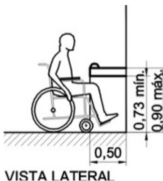
Área de Aproximação Bebedouro - Exemplo NBR9050:2004
