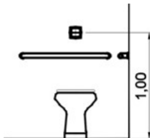
Bacia Sanitária - Altura de acionamento da descarga Exemplo NBR9050:2004
