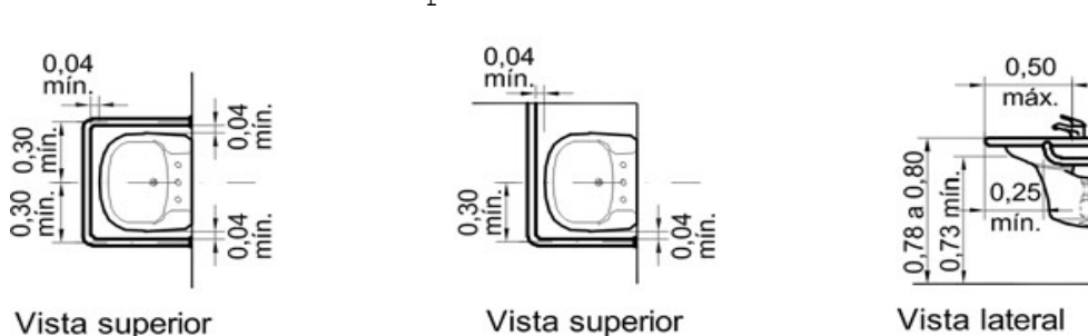
Barras de apoio em Lavatórios Embutidos em Bancadas Exemplo NBR9050:2004
