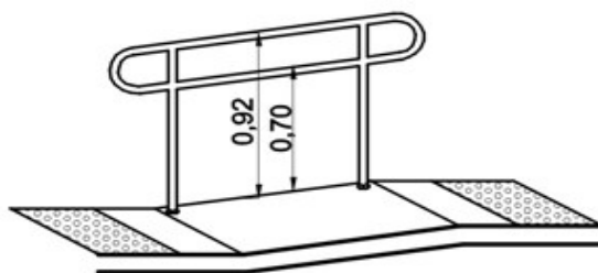
Corrimãos em rampas - Exemplo NBR9050:2004
