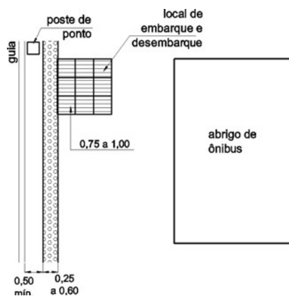
Sinalização de Ponto de Ônibus - Exemplo NBR9050:2004
