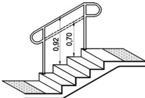
Corrimãos em degraus - Exemplo NBR9050:2004
