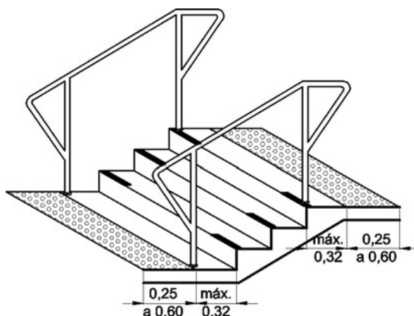
Sinalização tátil de alerta em escadas Exemplo NBR9050:2004
