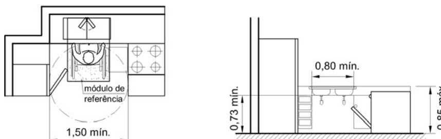
Copas, cozinhas ou similares - exemplos NBR9050:2004
