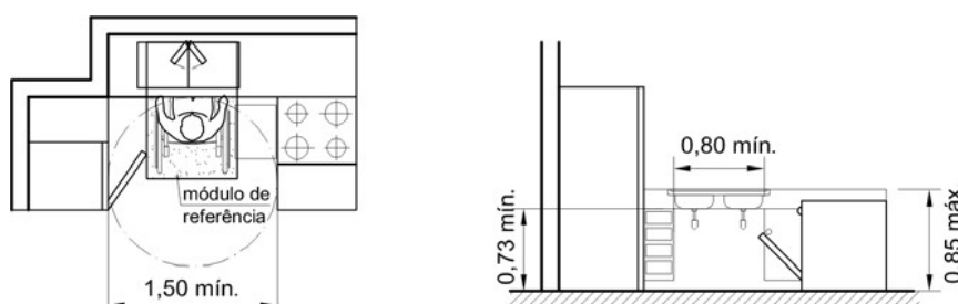
Copas, cozinhas ou similares - exemplos NBR9050:2004
