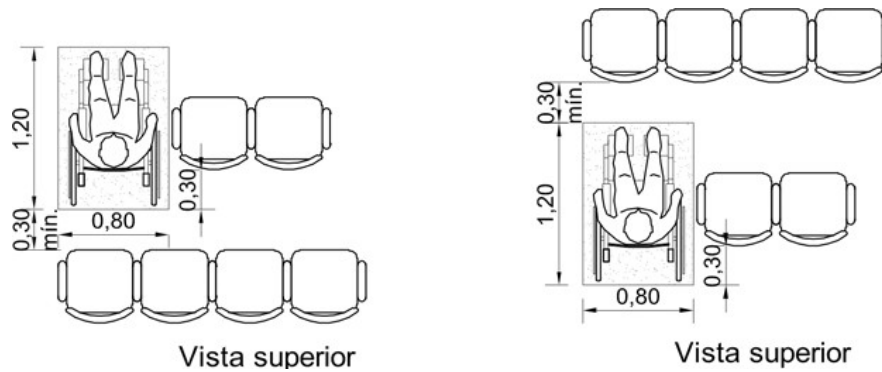
Espaço P.C.R. 1 a Fileira
