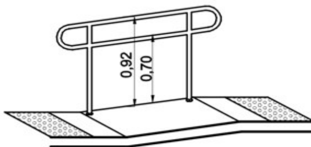
Corrimãos em rampas - Exemplo NBR9050:2004
