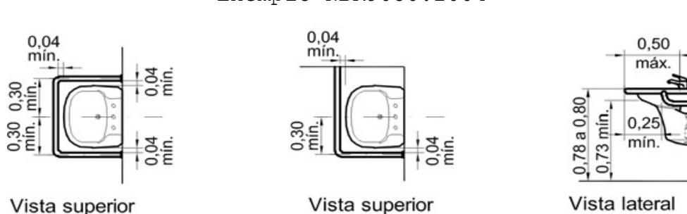
Barras de apoio em Lavatórios Embutidos em Bancadas Exemplo NBR9050:2004
