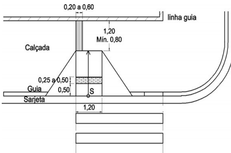
Vista superior
