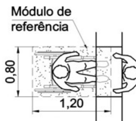
Vista Superior
