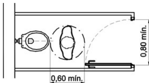
Boxe para bacia sanitária comum - Exemplo NBR9050:2004
