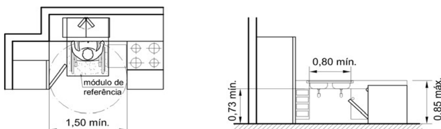
Copas / Cozinhas - Exemplo NBR9050:2004
