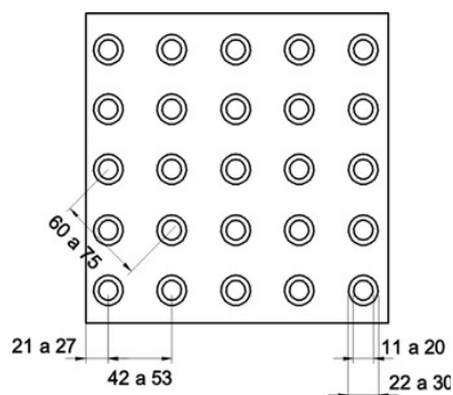
Sinalização Tátil de Alerta - Modulação do Piso Exemplo NBR9050:2004
