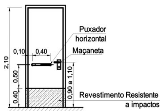
Porta com revestimento e puxador horizontal Exemplo NBR9050:2004
