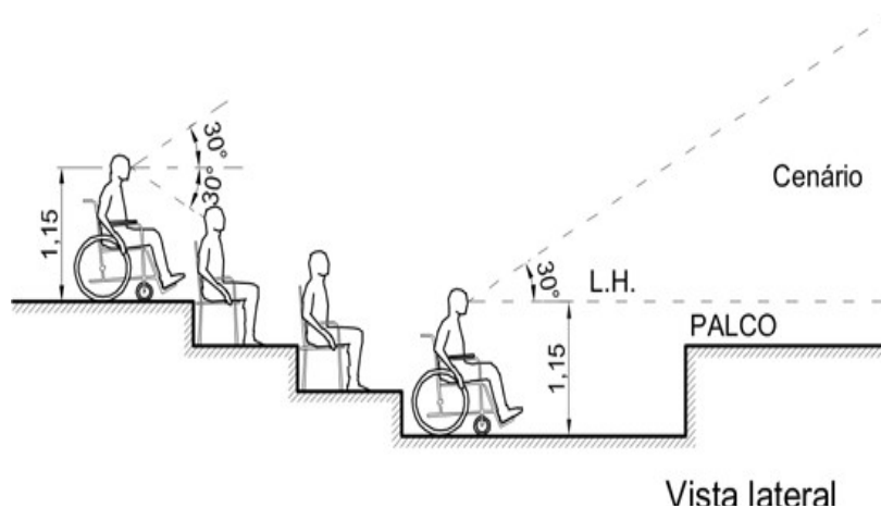
Ângulo Visual dos Espaços para P.C.R. em Auditórios Exemplo NBR9050:2004
