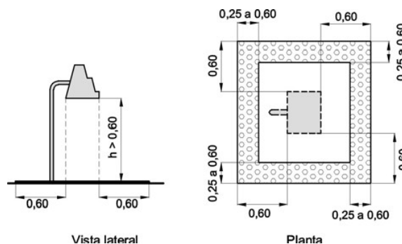
Sinalização tátil de alerta em obstáculos suspensos Exemplo NBR9050:2004
